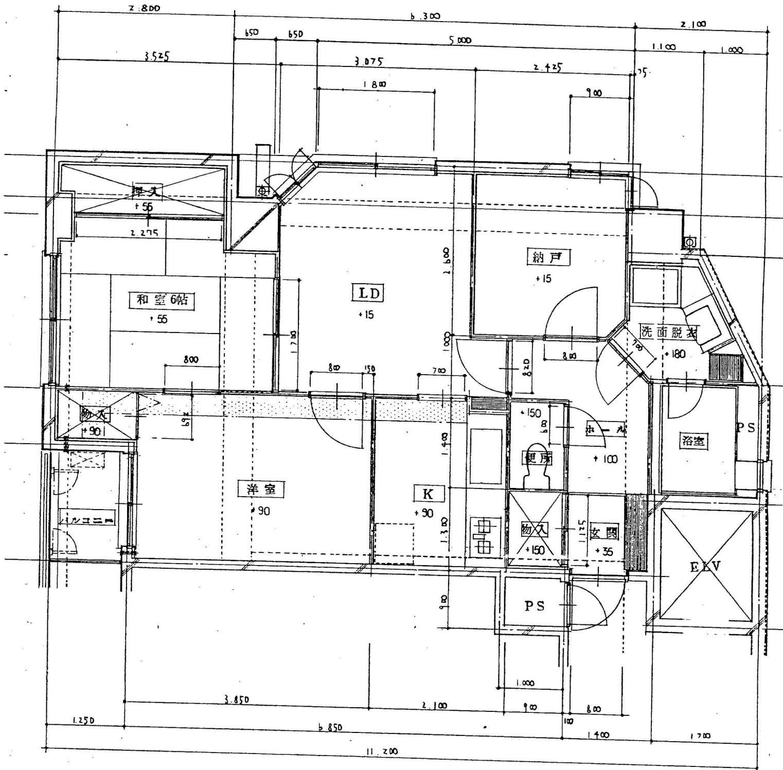
A タイプ 平面詳細図 1:50
